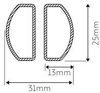
PROFILÉS INTERMÉDIAIRES
